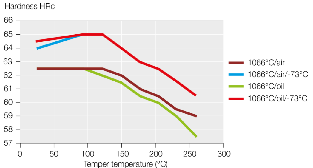
Abbildung 3 Anlassen Schaubild Temper hardness
