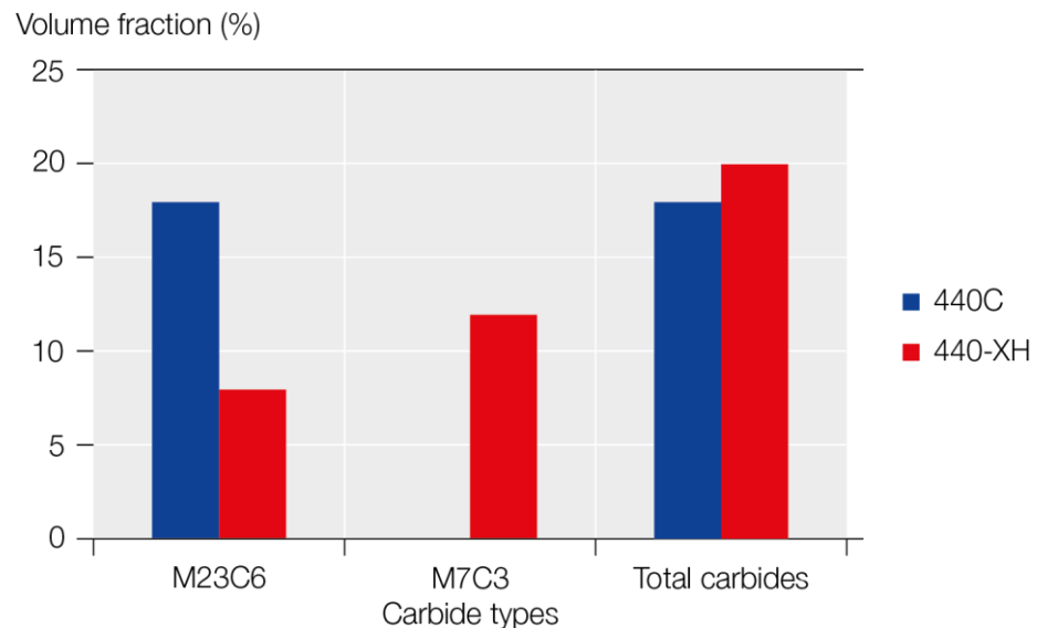
Abbildung 5 Karbidtypen
