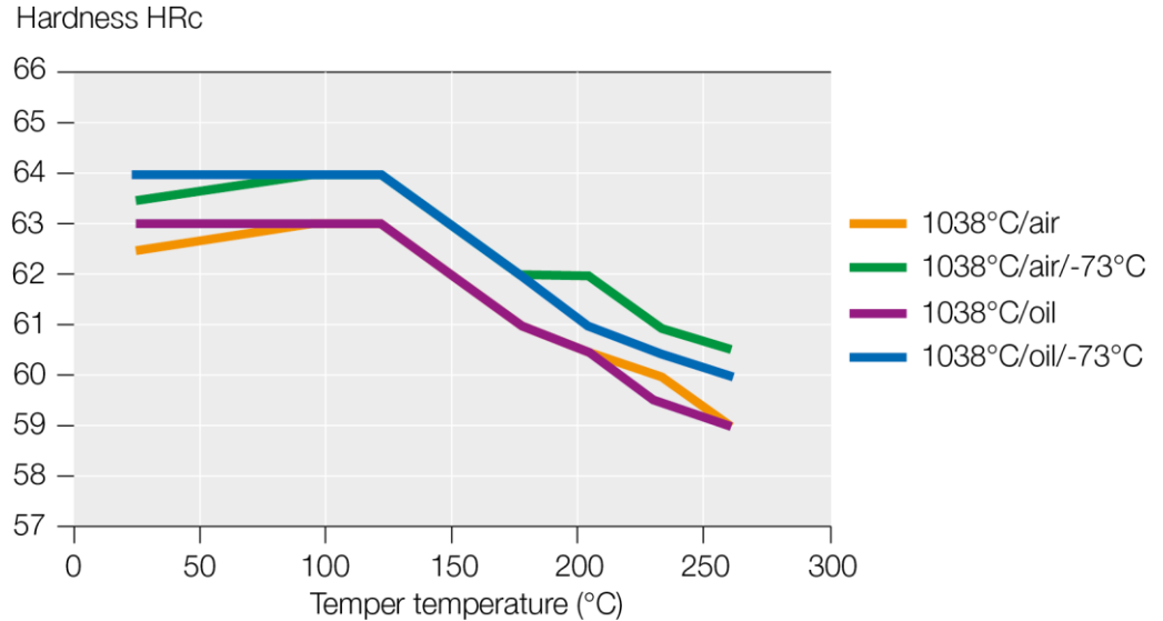
Abbildung 2 Anlassen Schaubild Temper hardness Quenching at 1038°C
