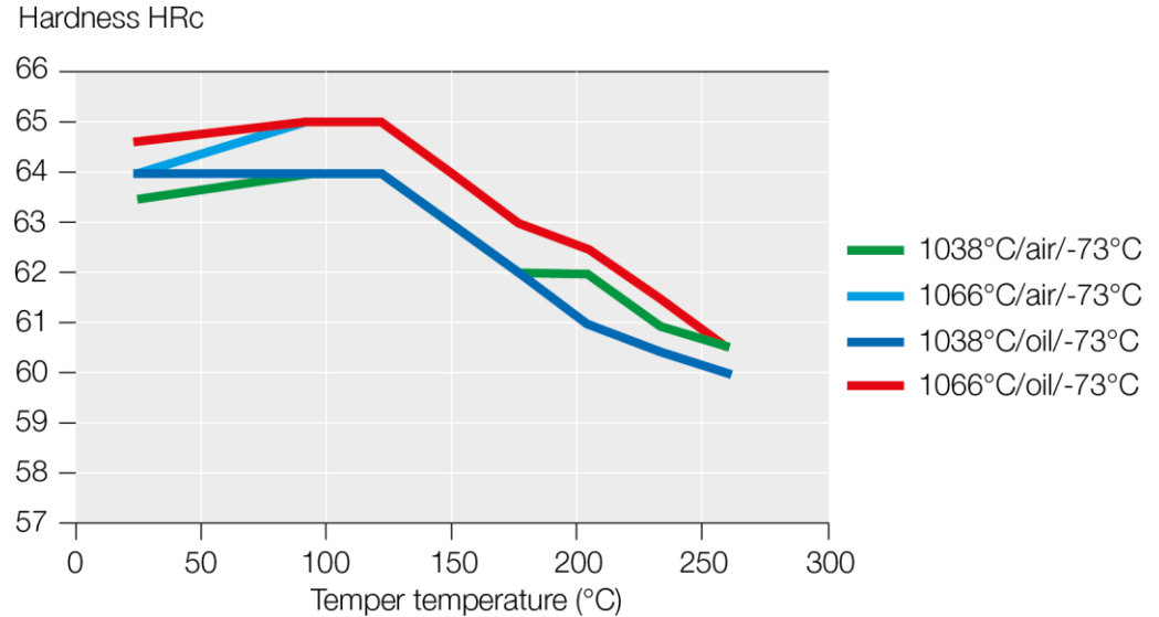
Abbildung 4 Anlassen Schaubild Temper hardness
