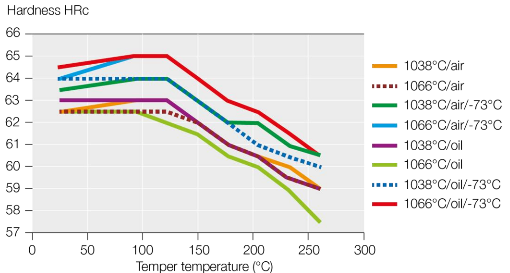
Abbildung 1 Anlassen Schaubild
